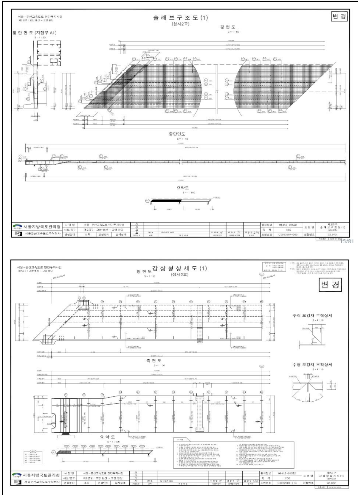
【그림 26.1.6】 바닥판하면 구조도, 강상형 상세도
