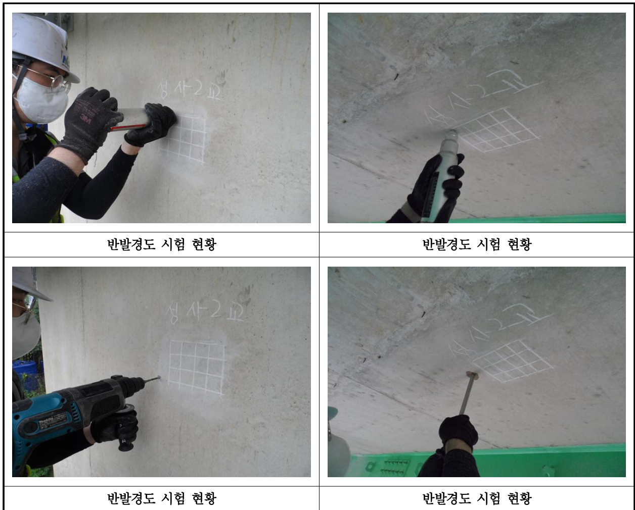
【사진 26.4.1】 콘크리트 내구성조사 현황
